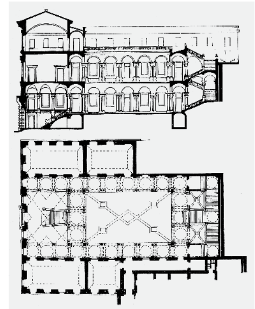
84 Genua, Palazzo dell'Università. Längsschnitt und Grundriss
